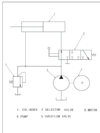
Hydraulische schema
